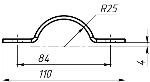
Поз.5 (Полухомут)
