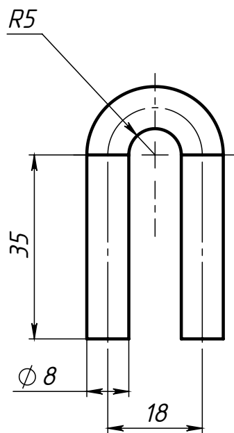
Поз.2 (Ушко) 1:1
