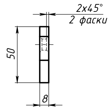
Поз.1 (Проушина)
