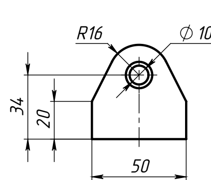
Поз.1 (Проушина)
