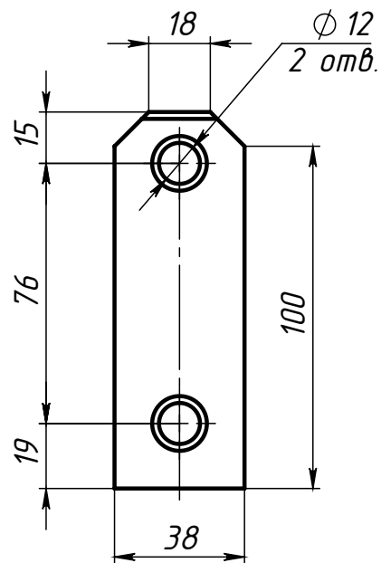
Поз.4 (Серьга)
