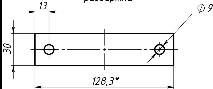
Поз.5 (Полухомут) развертка
