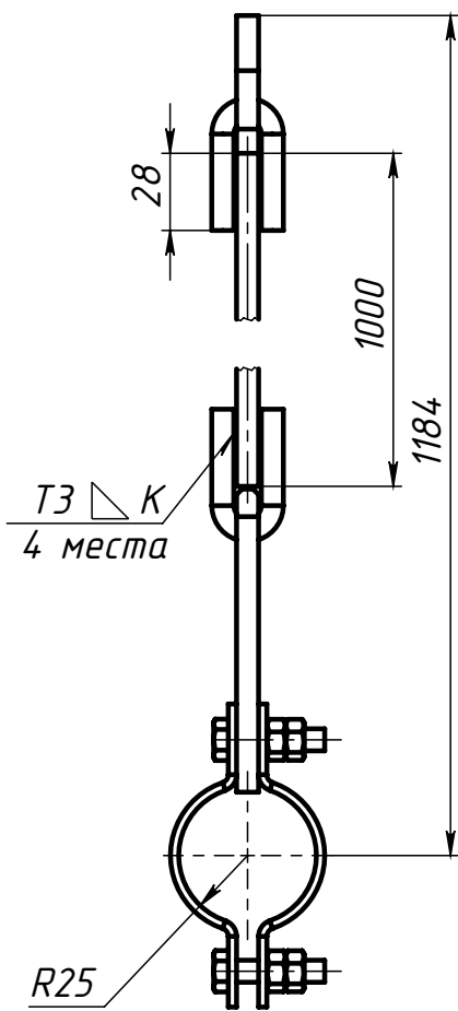
Поз.5 (Полухомут)
